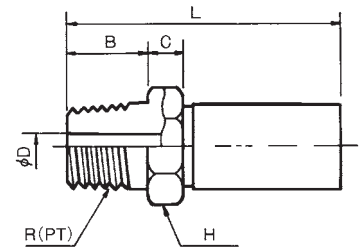
管用テーパおねじ
