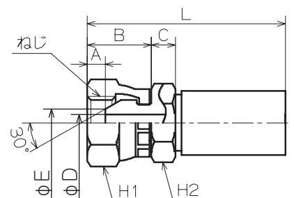
管平行めねじ (おすシート)
