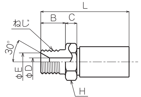
管平行おねじ
