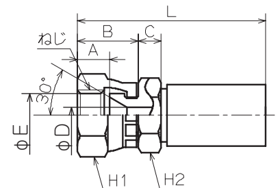
管平行めねじ (めすシート)
