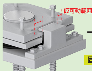
架設時(仮可動)
