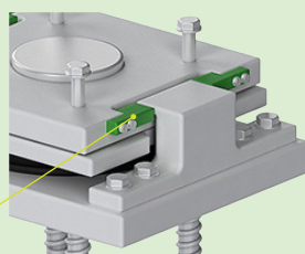
架設完了時(固定)
