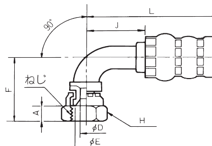
90° ベンドフィッティング (めすシート)
