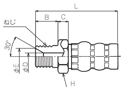
管用平行ネジ
