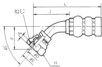
45° ベンドフィッティング (おすシート)
