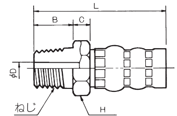
管用テーパーおねじ
