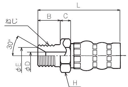
管用平行おねじ
