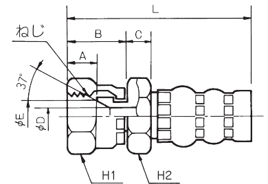
UNFめねじ (めすシート)
