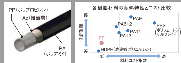
BEV冷却配管用樹脂チューブ
